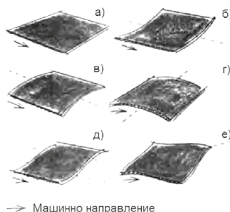
Фиг. 1 Видове изкорубване на вълнообразния картон:
